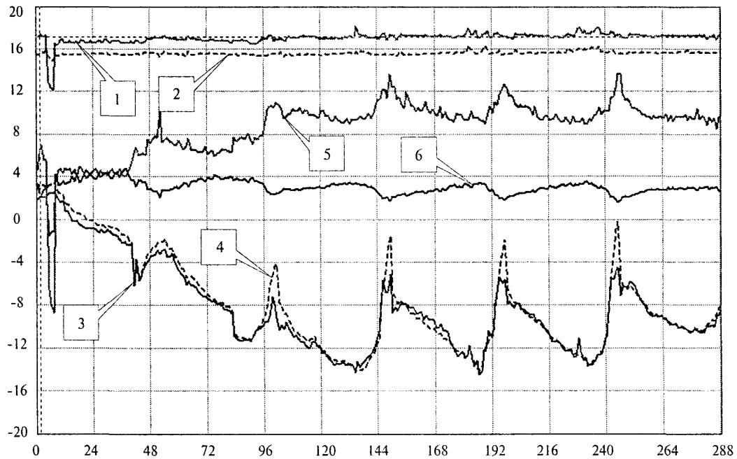
Рис. 3. Графики регистрируемых величин, по оси абсцисс отложены точки измерения с интервалом 30 мин, по оси ординат — температура (°C), плотность теплового потока (Вт/м 2 ), сопротивление теплопередаче (м 2 ·°C/Вт)
