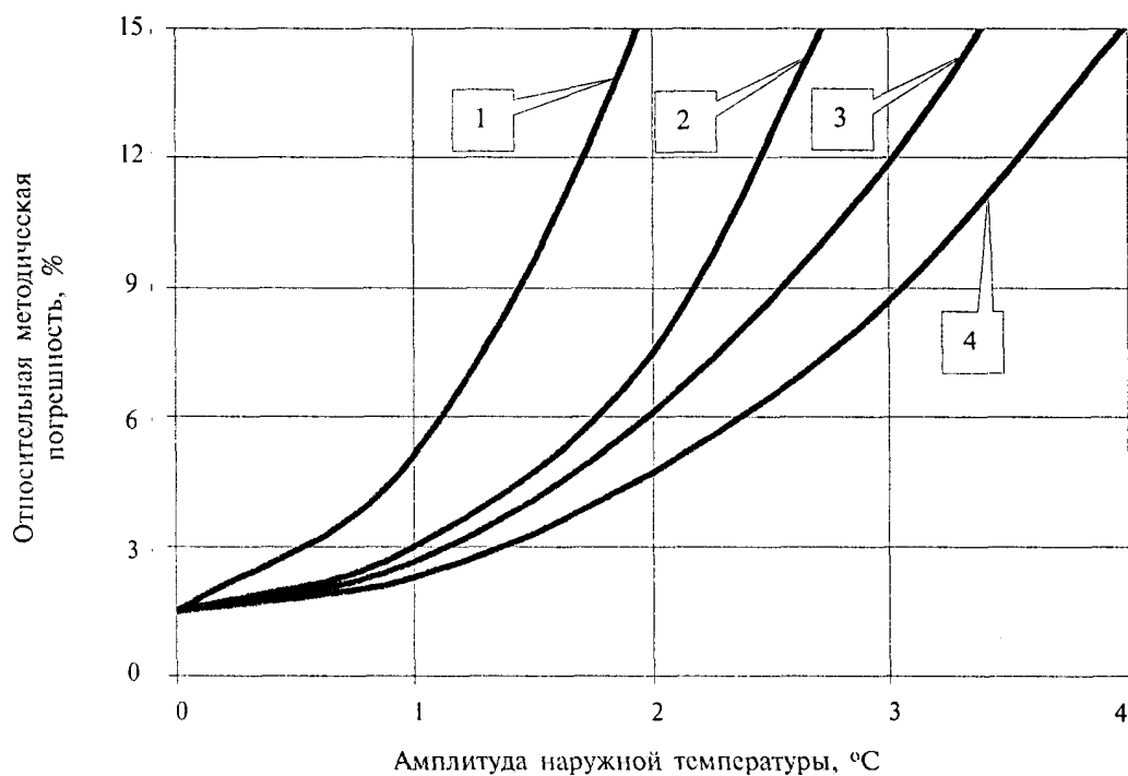
Рис. 2. Графики к определению методической погрешности вычисления R_T при измерении теплового потока на внутренней поверхности 1 - при \tau_e - \tau_n = 20 °C; 2 — при \tau_e - \tau_n = 30 °C; 3 — при \tau_e - \tau_n = 40 °C; 4 — при \tau_e - \tau_n = 50 °C
