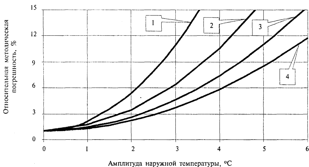
Рис. 1. Графики к определению методической погрешности вычисления R_T при измерении теплового потока на наружной поверхности 1 — при \tau_{\theta} - \tau_n = 20 °С; 2 — при \tau_{\theta} - \tau_n = 30 °С; 3 — при \tau_{\theta} - \tau_n = 40 °С; 4 — при \tau_{\theta} - \tau_n = 50 °С
